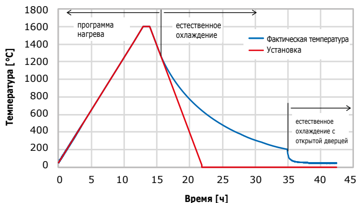
Режим спекания в печи HTF 18/64
